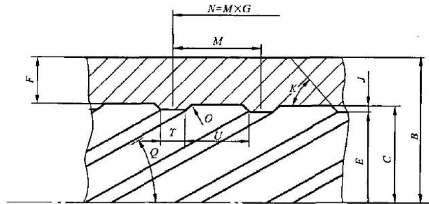
Lognitudinal
